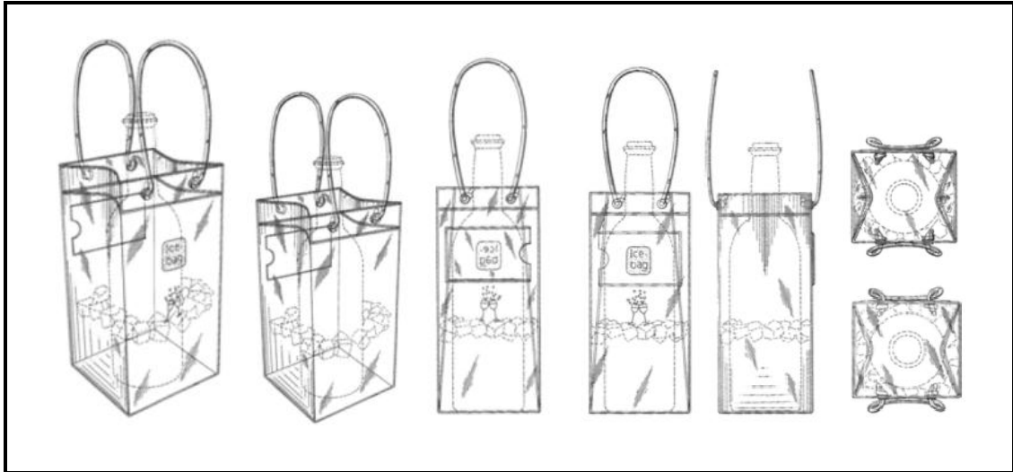
圖2 Gimex的 RCD 000616057-0001的Ice Bag設計
